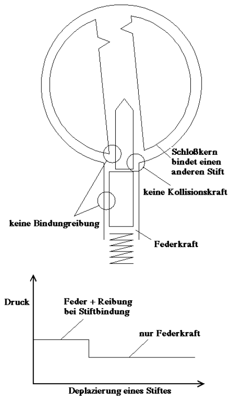
Abbildung 9.3: Dünner Kernstift
