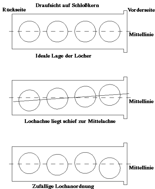
Abbildung 6.2: Ausrüstung der Löcher im Schloßkern
