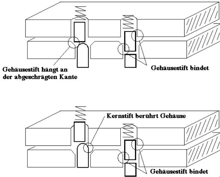
Abbildung 9.4: Abgeschrägte Schloßkernlöcher und abgerundete Kernstifte
