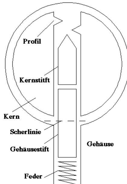
Abbildung 5.1: Das Stift-Säulen-Modell
