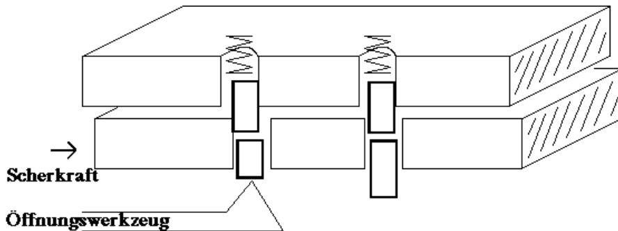
Abbildung 4.2: Das Öffnungswerkzeug drückt den linken Kernstift
